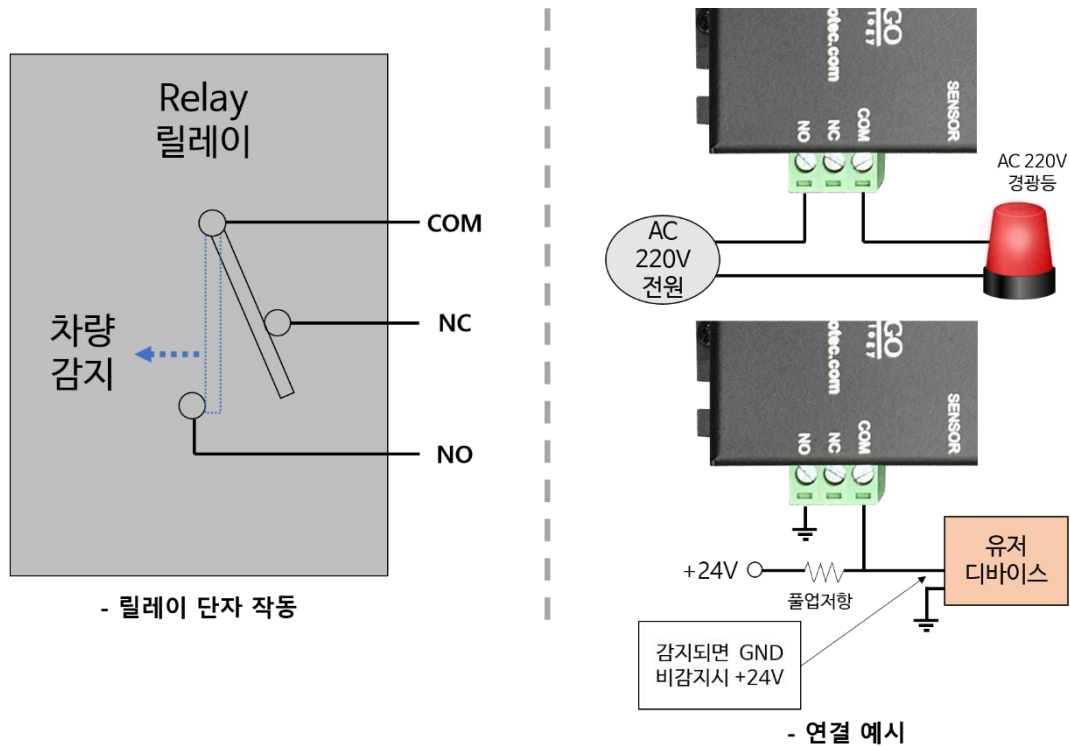
그림 5. 외부기기의 연결(예시)
