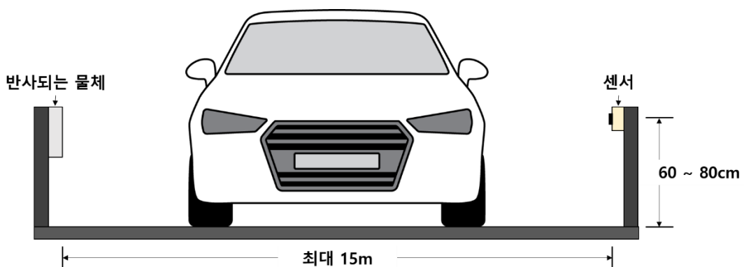
그림 1. 차량검출센서 CARDET-LD의 설치 1번 예시
