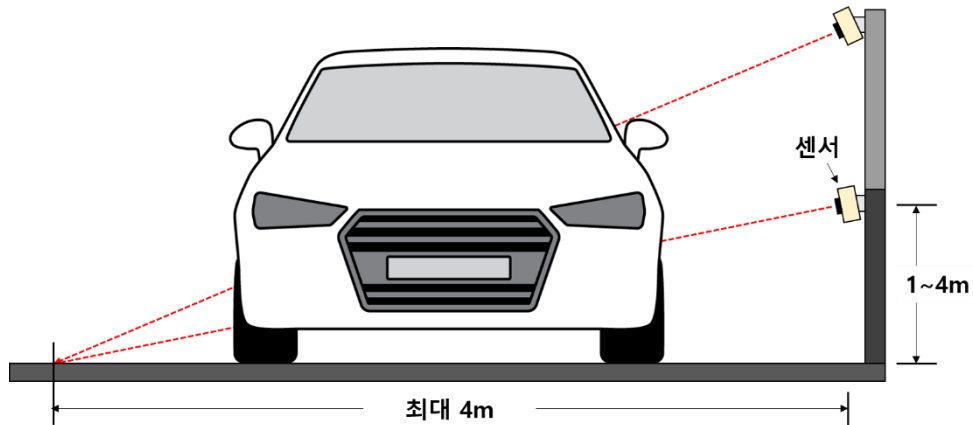
그림 2. 차량검출센서 CARDET-LD의 설치 2번 예시
